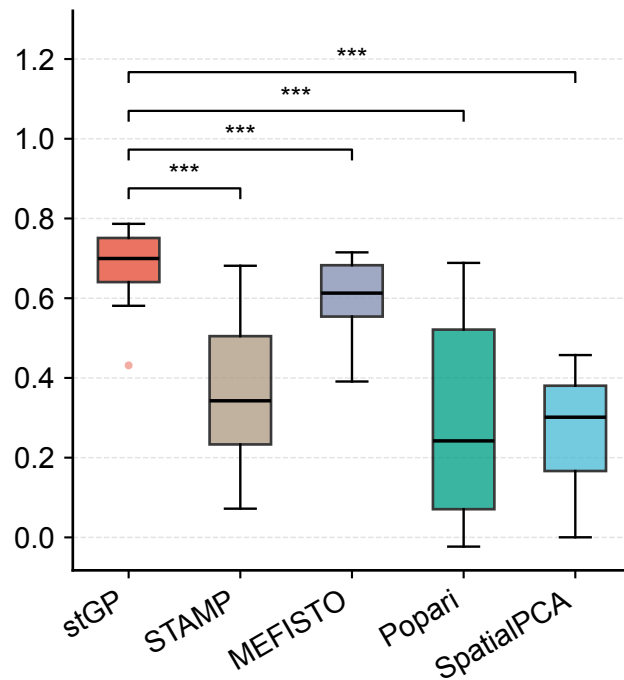
L4 ( RORB )
